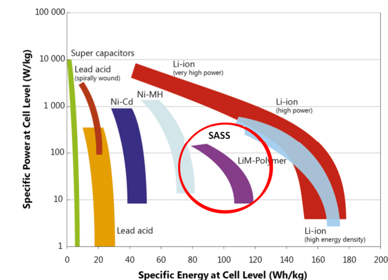
Abbildung 10 – Energie- und Leistungskurve verschiedener Batterietechnologien
