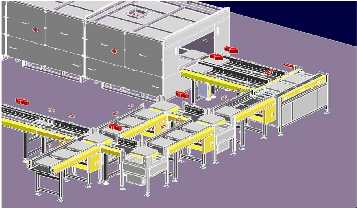
Abbildung 22 – Altech Vorschubofen von Riedhammer
