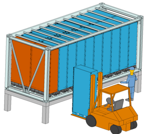
Abbildung 26 – GridPack-Montage
