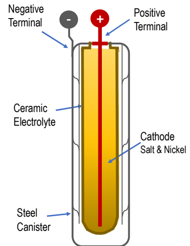
Abbildung 7 – Komponenten der CERENERGY®-Batterie
