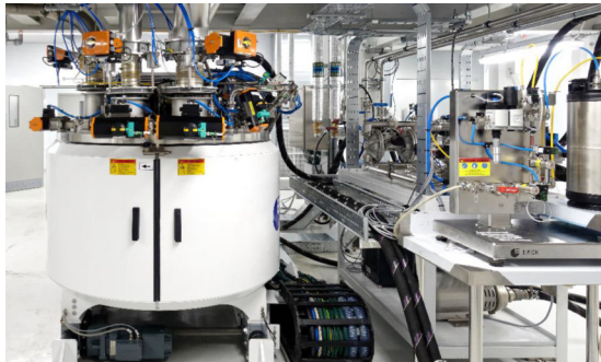
Abbildung 20 - Eirich Prozessanlagen
