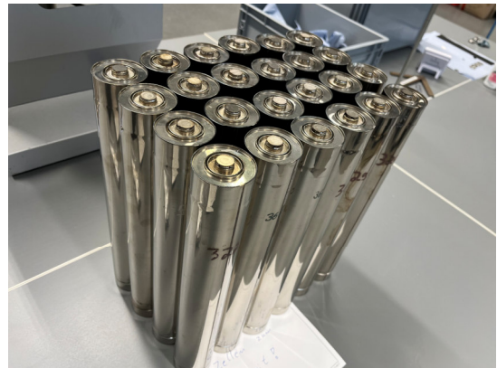
Abbildung 11 – CERENERGY® Prototypenzellen
