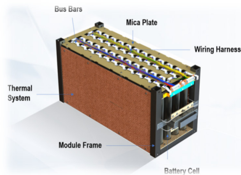
Abbildung 13 – CERENERGY®-Batteriemodul
