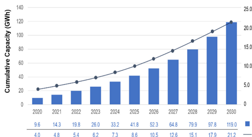
Abbildung 16 – globale Marktentwicklung für Energiespeicher, Quelle: Bloomberg NEF
