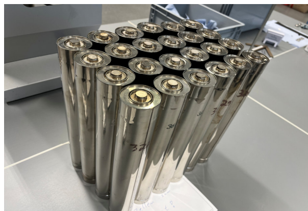
Abbildung 35 – Fertiggestellte Prototypenzellen bereit für den Teststand
