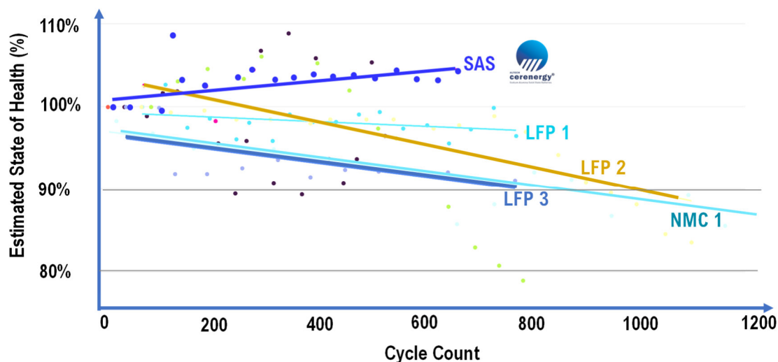
Abbildung 2 - Prüfung der Lebensdauer verschiedener Batterien, einschließlich Batterien des Typs CERENERGY® Source: ITP Renewables Public Report 11 Lithium-ion Battery Testing Sep 2021
