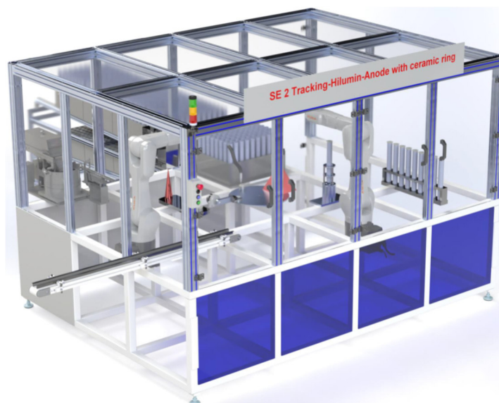
Abbildung 23 – Anlage für Thermokompressionsklebverfahren
