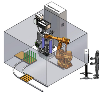
Abbildung 21 - Freys Isostatische Presseeinheit
