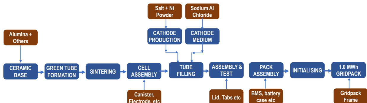
Abbildung 18 – Schematisches Prozessschaubild
